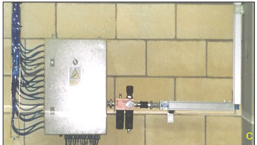
C: Biogas (Spagna) - Vista generale con linea di alimentazione (HBS25), filtro e regolazione ed uscite.
