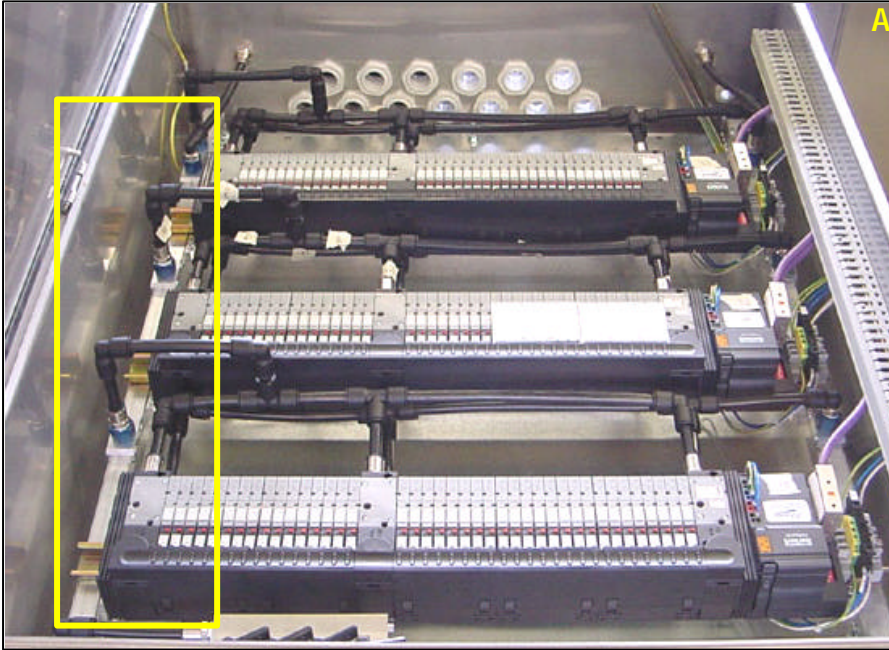
A,B: Ebora (Olanda) - Collettori modulare (AP 20) alimenta un gruppo di elettrovalvole.
